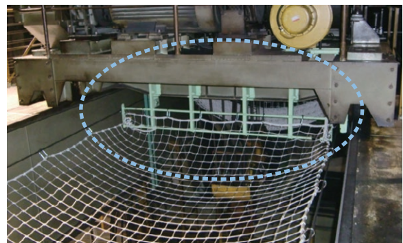
トロリ側：安全ネット干渉防止柵
