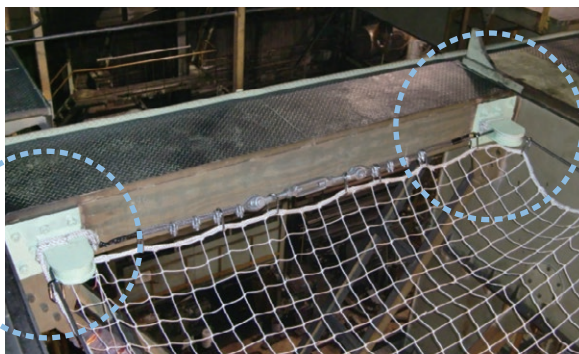
サドル側：安全ネット用ワイヤ支持ブラケット
