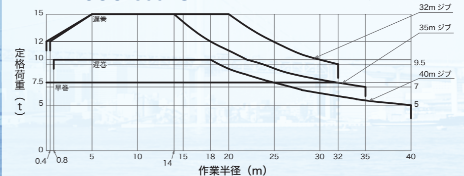
JCC-300VS サステナ 定格荷重曲線表
