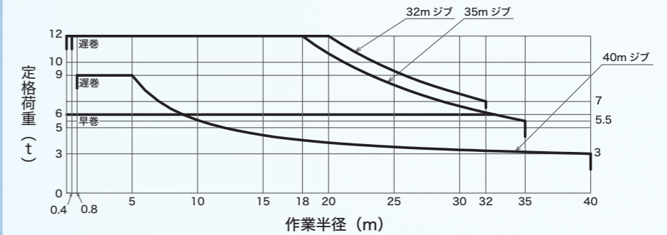
JCC-230II サステナ 定格荷重曲線表
