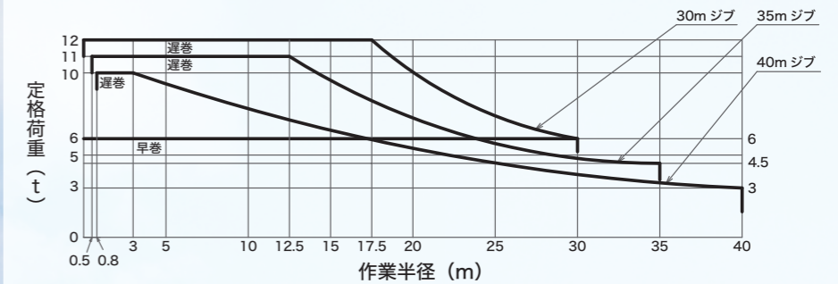
JCC-180U サステナ 定格荷重曲線表
